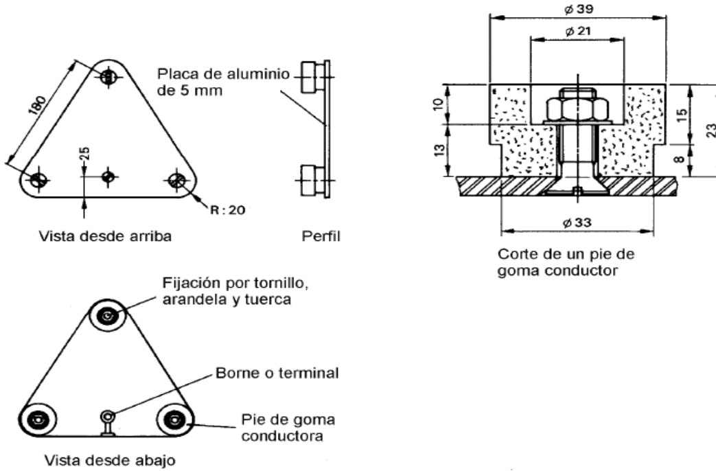
Figura 19.1.1 – Electrodo de ensayo 1
