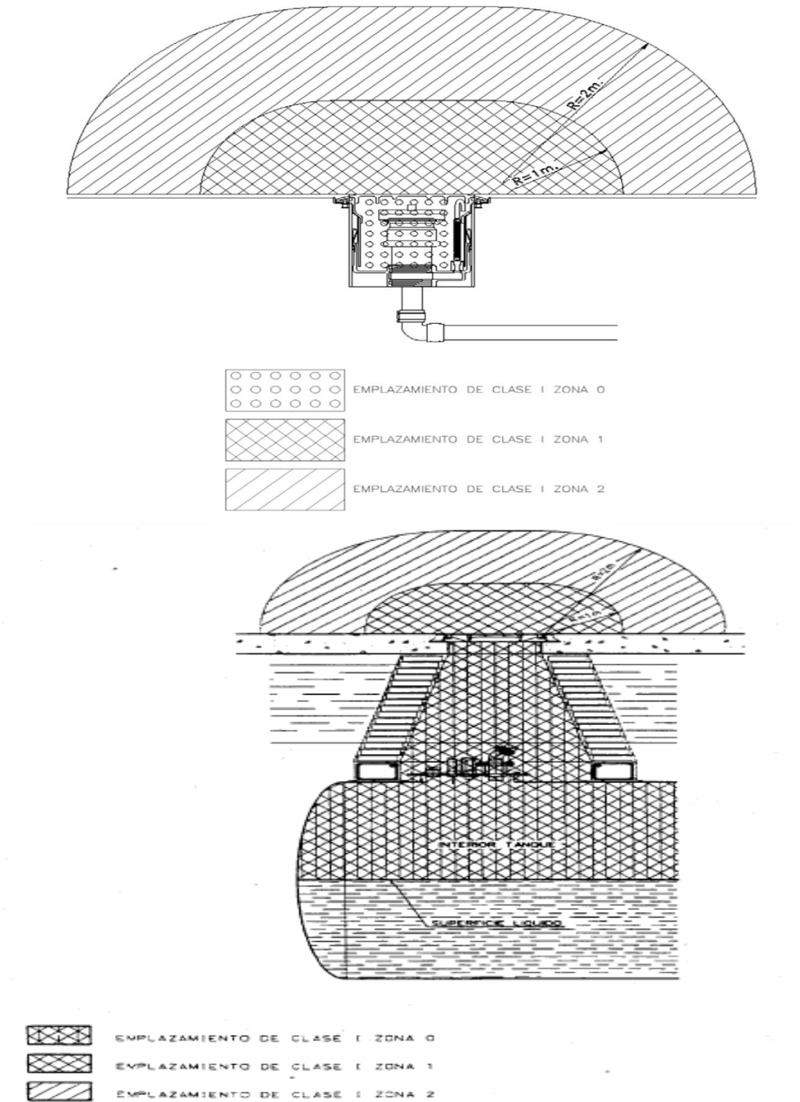
FIG. 5 DETALLES TÍPICOS DE LA CLASIFICACIÓN EN ARQUETAS O TAPA DE SEGURIDAD.
