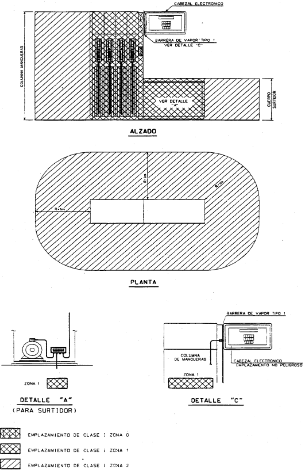
FIG. 2 SURTIDOR CON CABEZAL ELECTRÓNICO ELEVADO Y ADOSADO A LA COLUMNA DE MANGUERAS (BARRERA DE VAPOR TIPO 1)
