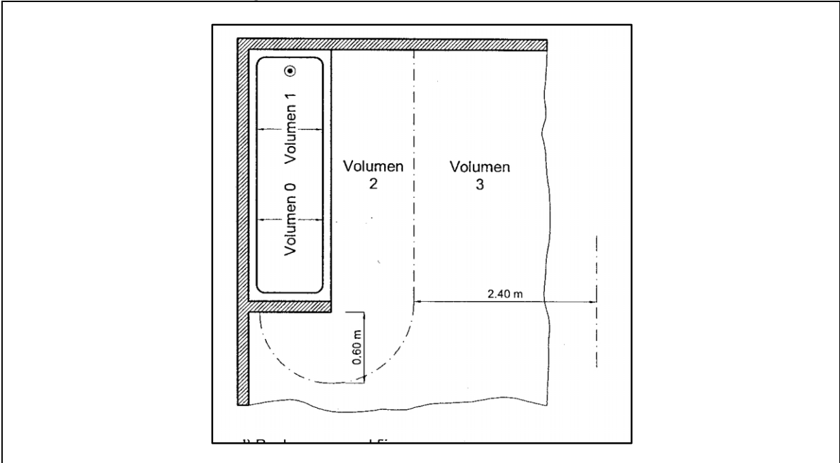
Figura 11.6.2 – BAÑERA CON PARED FIJA
