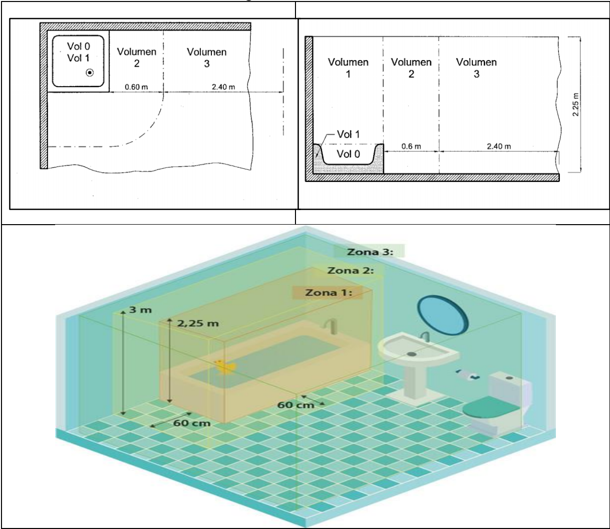
Figura 11.6.3 – DUCHA
