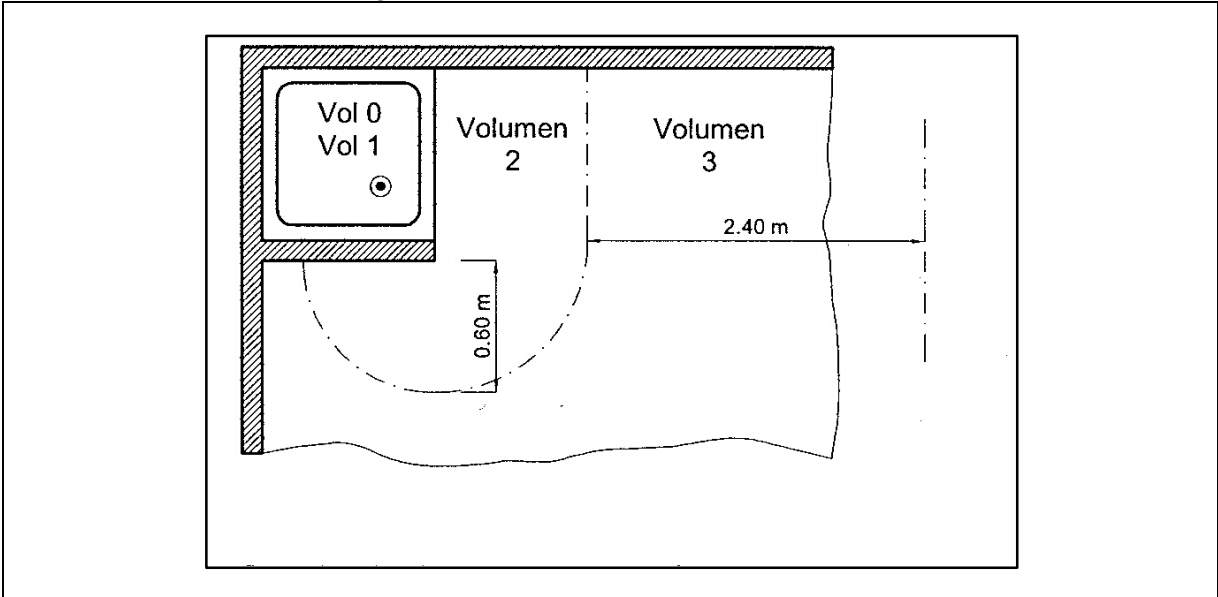
Figura 11.6.4 – DUCHA CON PARED FIJA
