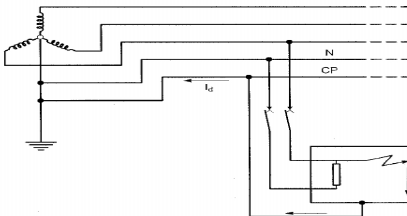
Figura 4. Esquema TN-S
