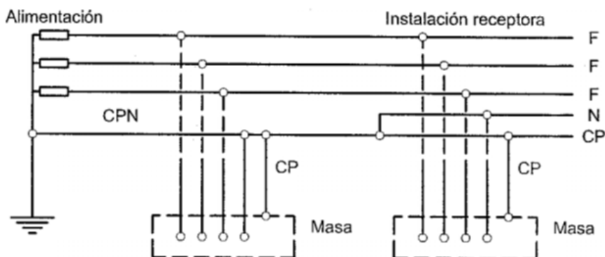
Figura 5.3 Esquema TN-C-S
