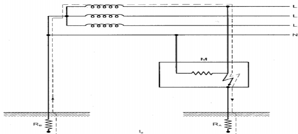
Figura 5 Esquema TT
