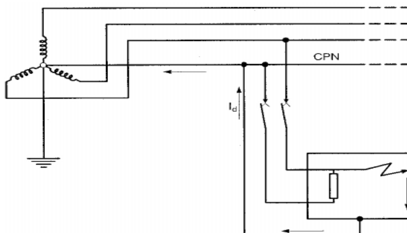
Figura 3. Esquema TN-C
