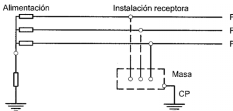
Figura 5.5 Esquema IT
