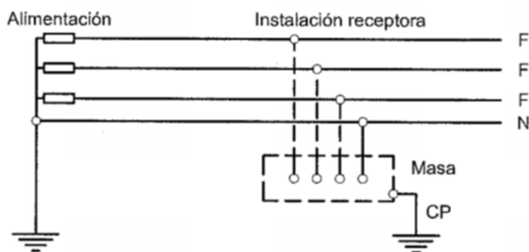
Figura 5.4 Esquema TT
