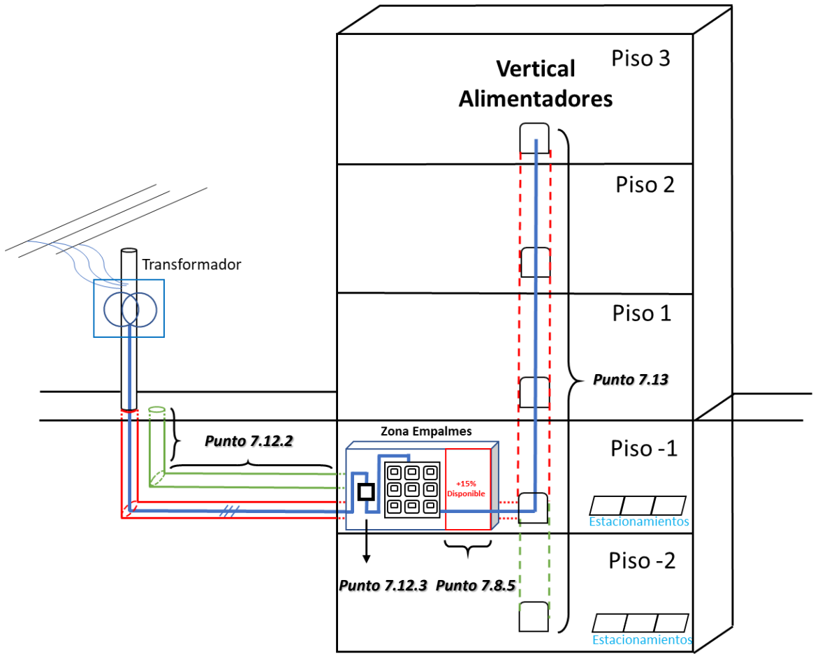
Fig. 1 Empalmes concentrados
